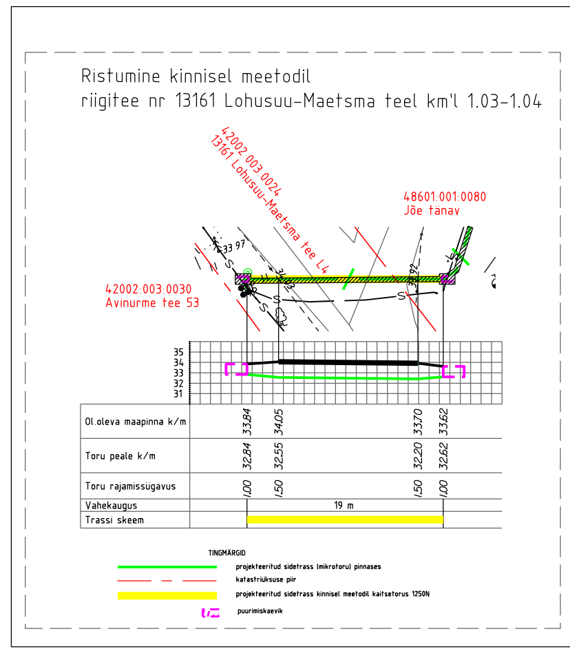
Väljavõte: Ristlõige 1:250
